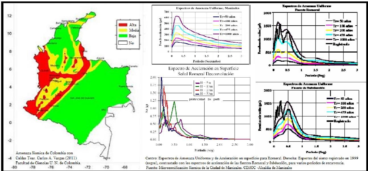
Imagen 41: Mapa no oficial de Amenaza Sísmica para Colombia según Carlos A. Vargas, en UN Periódico (2011), y Espectros de amenaza y de aceleración en la Microzonificación Sísmica para Manizales, del SIMOC (2002).
