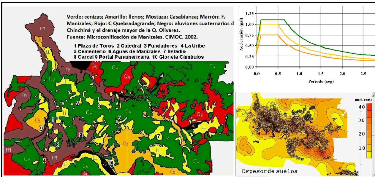
Imagen 42: Zonificación de Manizales según Cimoc (Der); y Espectros de diseño y espesores de suelos en Manizales (Der). Microzonificación Sísmica para Manizales, del SIMOC (2002).
