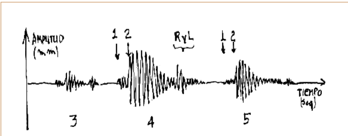
Figura 96. Sismograma. 1. Onda P, 2. Onda S, 3. Premonitor, 4. Paroxismo, 5. Répica. La diferencia de tiempo de arribo entre las ondas P y S, se mantiene en las tres sacudidas (3, 4 y 5), pues depende solo de la distancia Estación-Foco.
